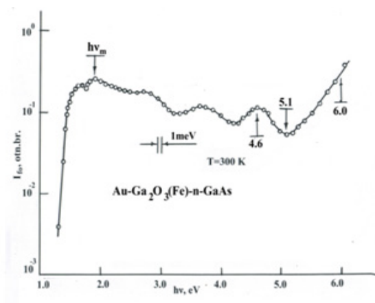
4-nji surat. Au-Ga 2 O 3 (Fe)-n-GaAs MDS nanogurluşyň fototogunyň spektri
