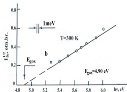
5-nji surat. I_0^{1/2} - h\nu koordinatada gurlan Au-Ga 2 O 3 (Fe)-n-GaAs MDS nanogurluşyň fototogunyň spektri
