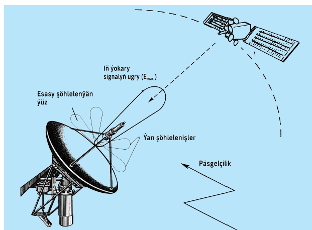
Antennanyň ugrukdyrys diagrammasy
